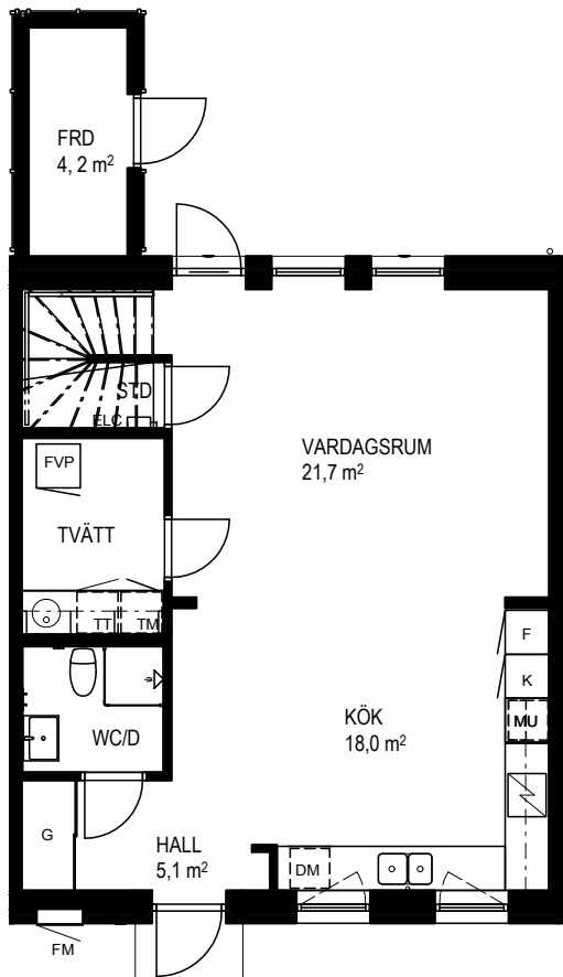
ENTRÉPLAN
