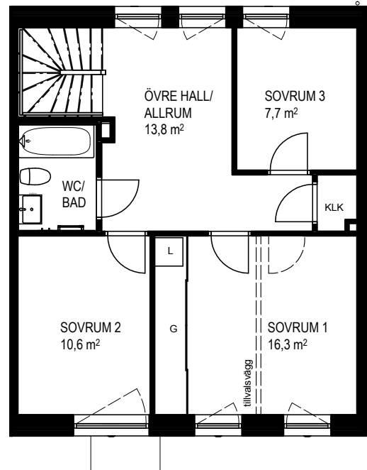
ÖVRE PLAN
