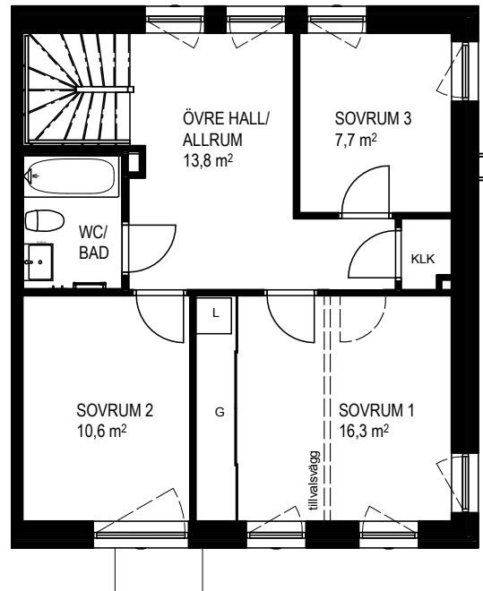
ÖVRE PLAN
