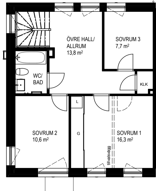
ÖVRE PLAN
