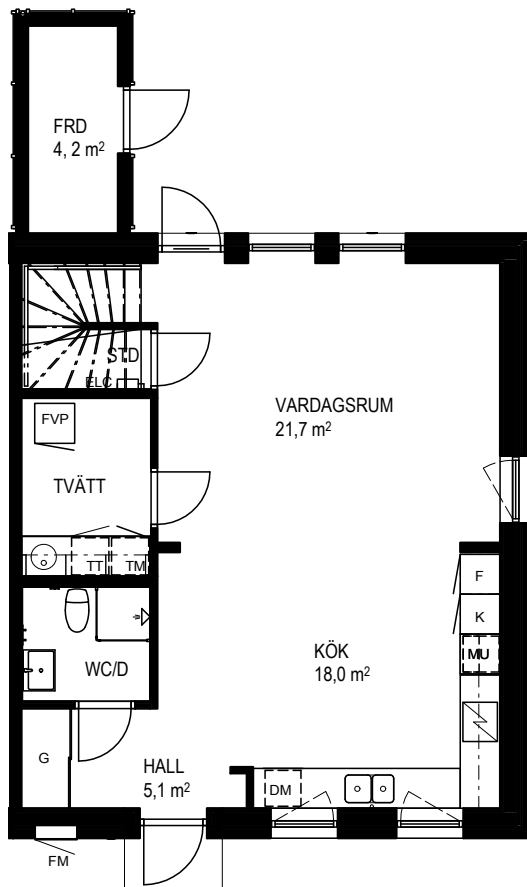
ENTRÉPLAN
