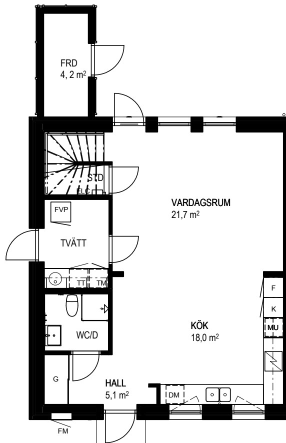
ENTRÉPLAN
