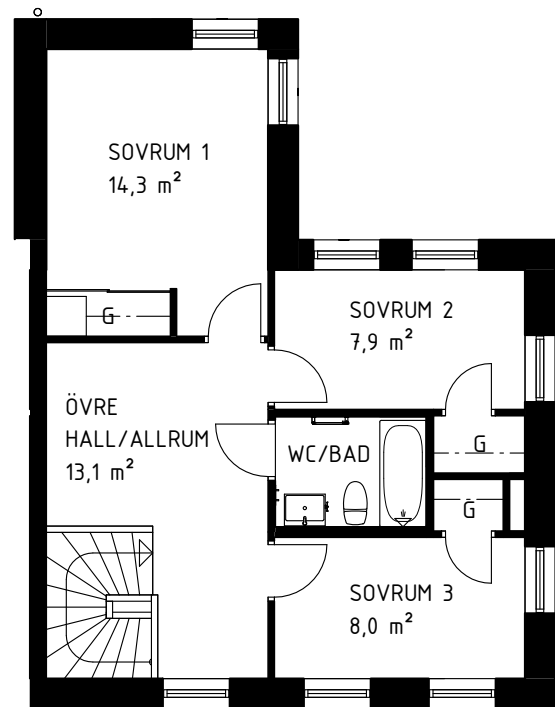
ÖVRE PLAN
