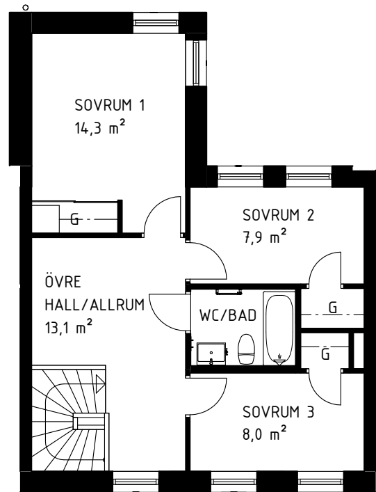
ÖVRE PLAN
