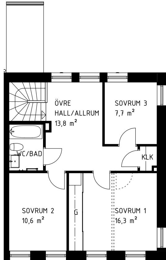
ÖVRE PLAN
