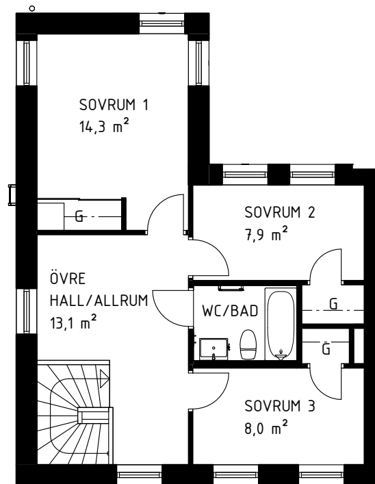
ÖVRE PLAN
