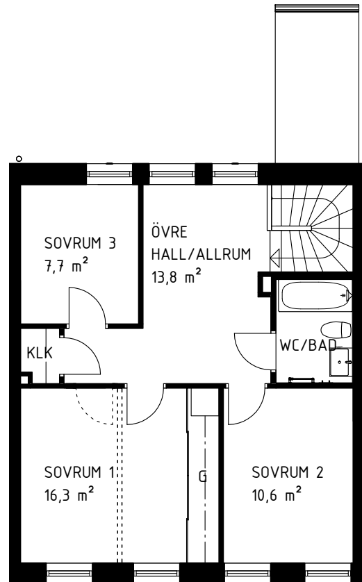
ÖVRE PLAN
