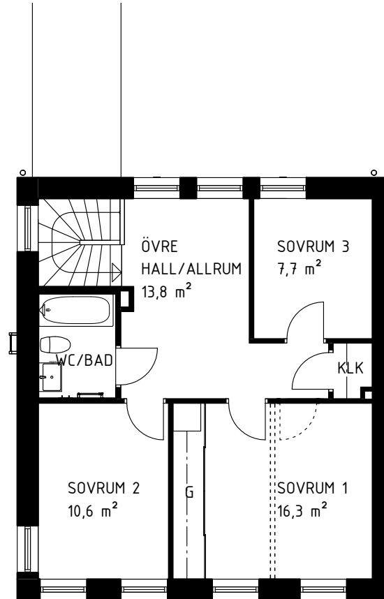
ÖVRE PLAN
