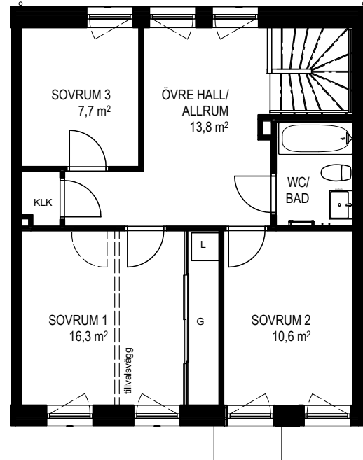
ÖVRE PLAN
