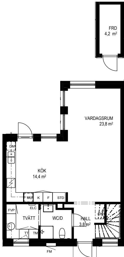
ENTRÉPLAN
