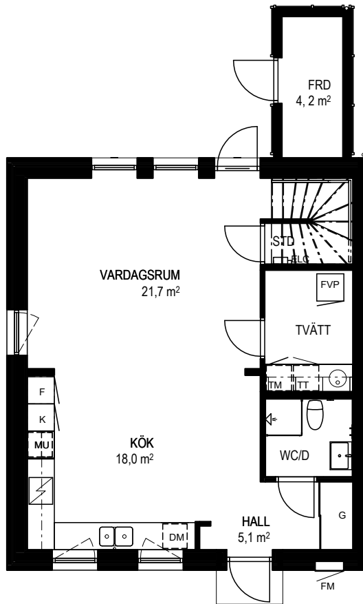
ENTRÉPLAN
