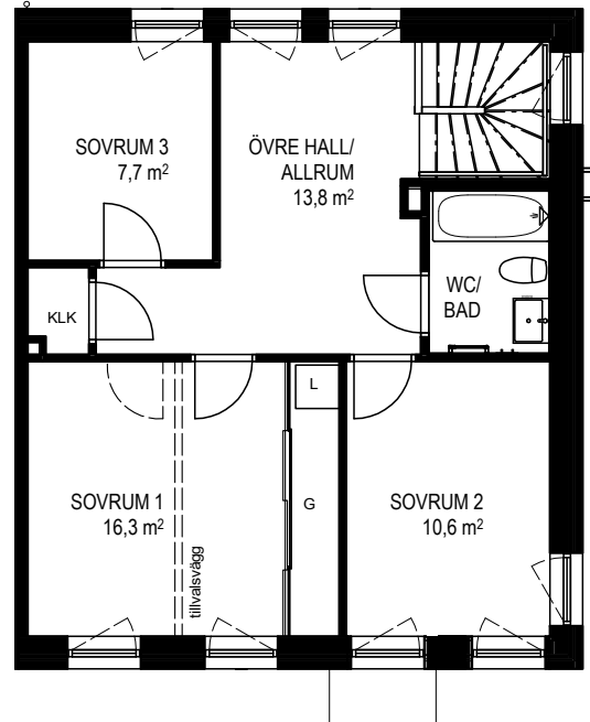
ÖVRE PLAN
