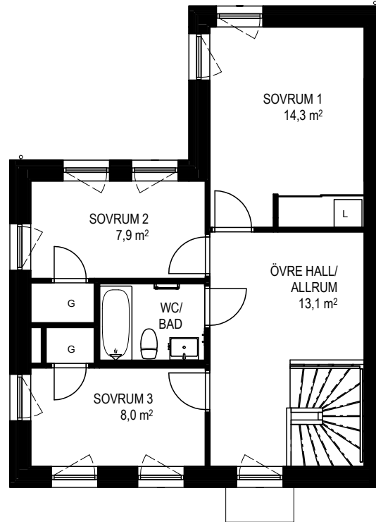
ÖVRE PLAN
