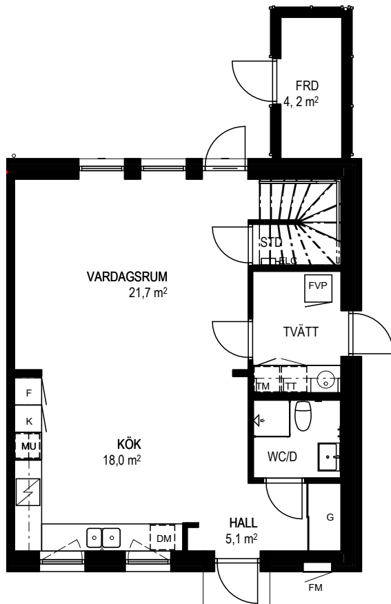
ENTRÉPLAN
