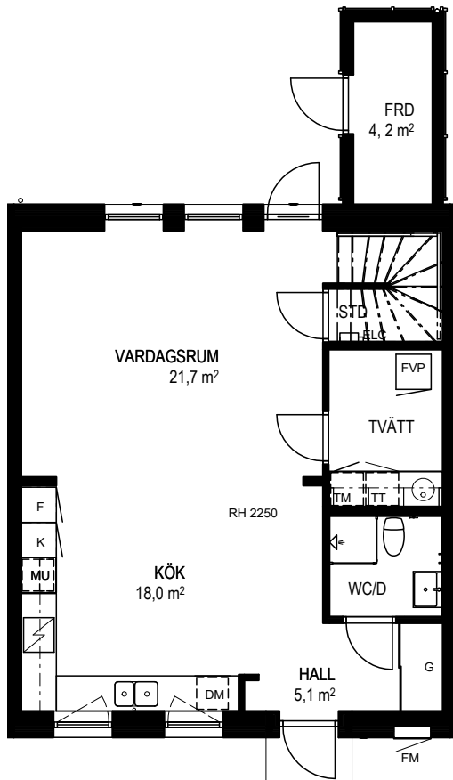
ENTRÉPLAN
