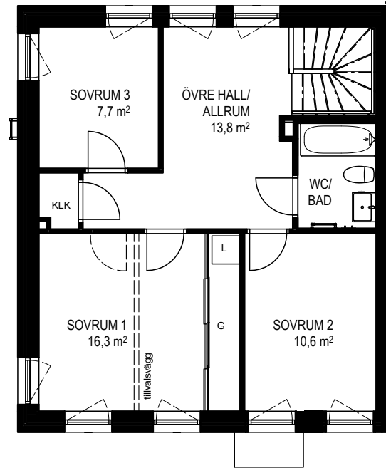
ÖVRE PLAN
