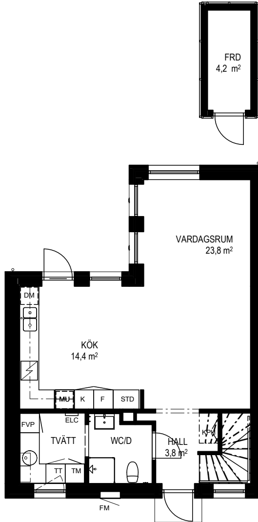
ENTRÉPLAN
