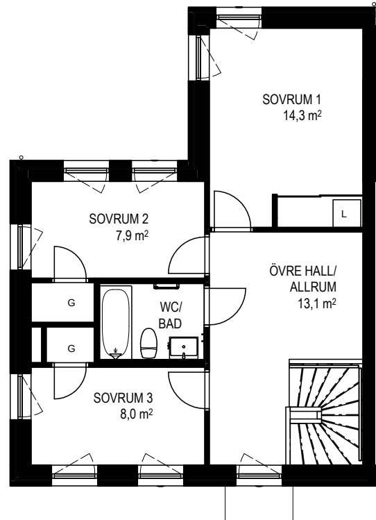
ÖVRE PLAN
