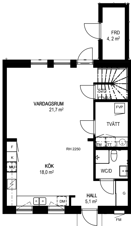
ENTRÉPLAN
