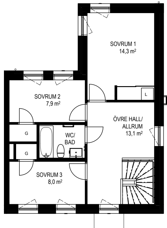
ÖVRE PLAN
