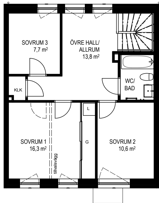
ÖVRE PLAN
