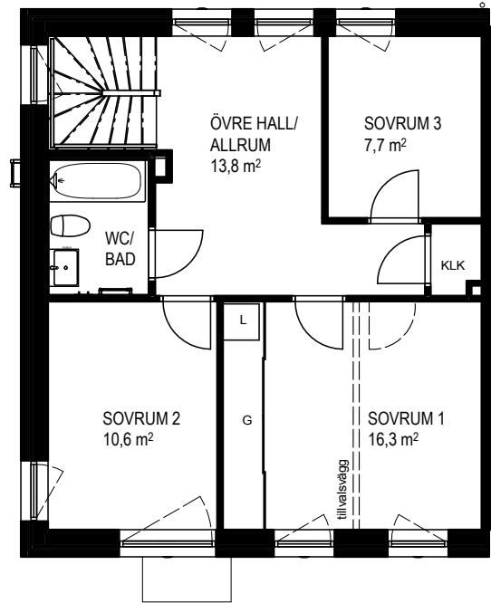
ÖVRE PLAN
