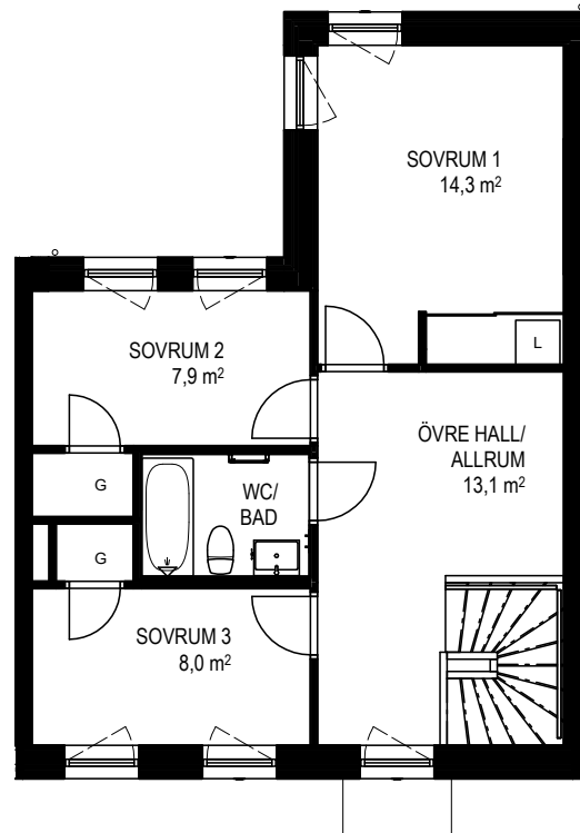
ÖVRE PLAN
