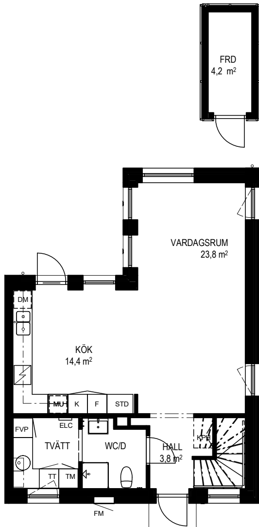
ENTRÉPLAN
